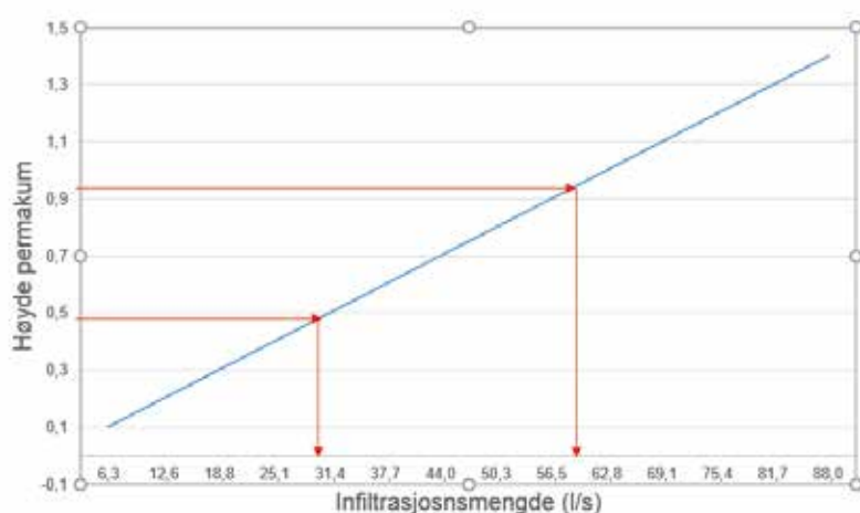
HØY INFILTRASJONSKAPASITET: Tetser av prototypen viste at en kunne "infiltrere" ut ca 20 l/s pr m 2 permeabelt lag
