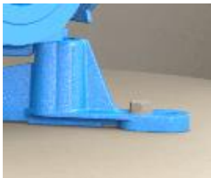
Betong/konsoll Hull i konsollfoten er laget for Bolt M24 C-C 550 og innstøpt bolt M27 C-C 620
