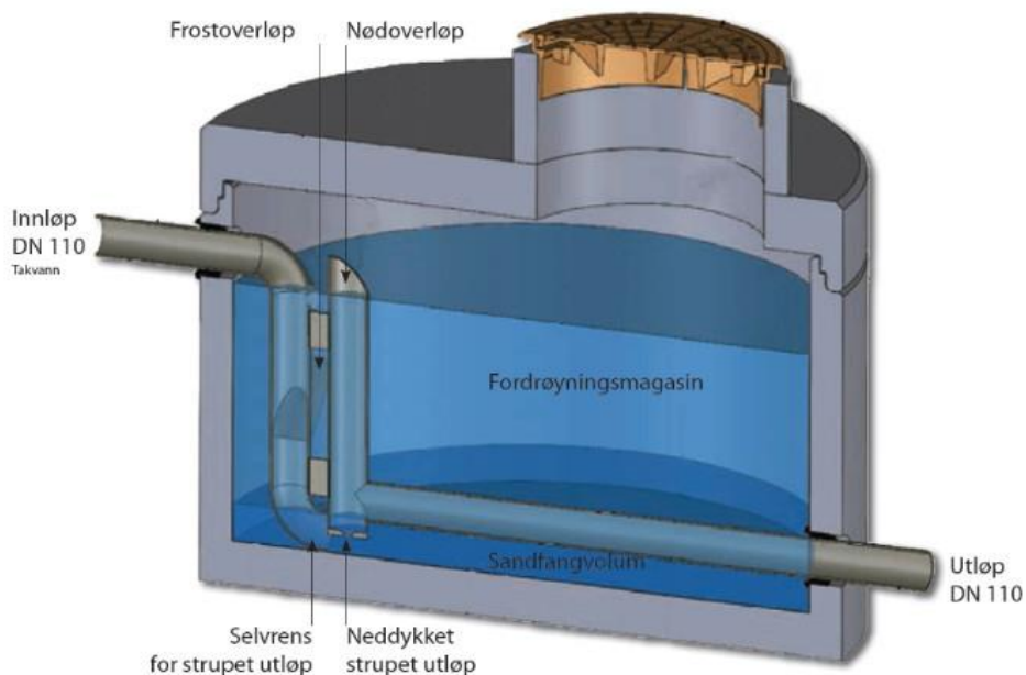
Principskisse - Oppbygning av LOD-kummen
